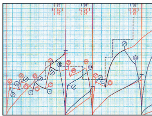
運転曲線
